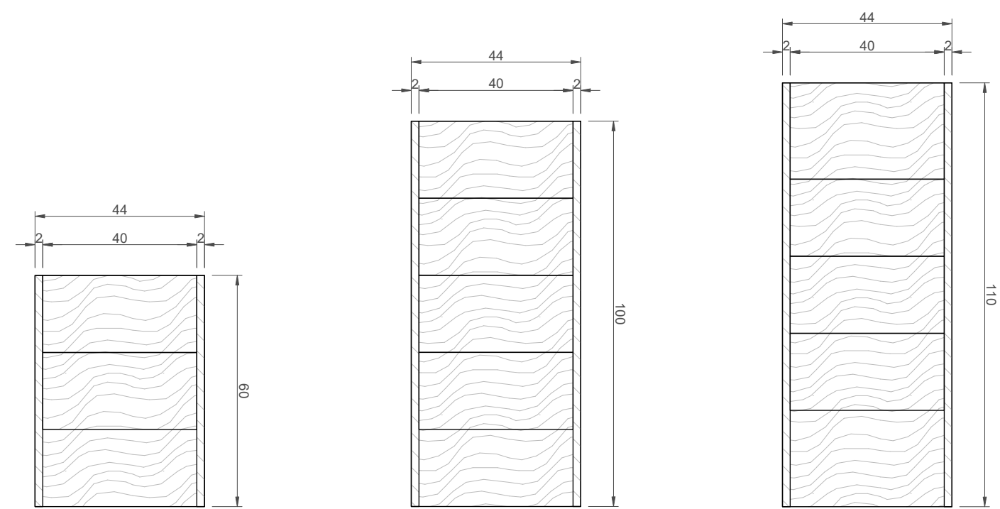
Höhe des Rahmens bei Drehflügeltüren und Standard-FIX
