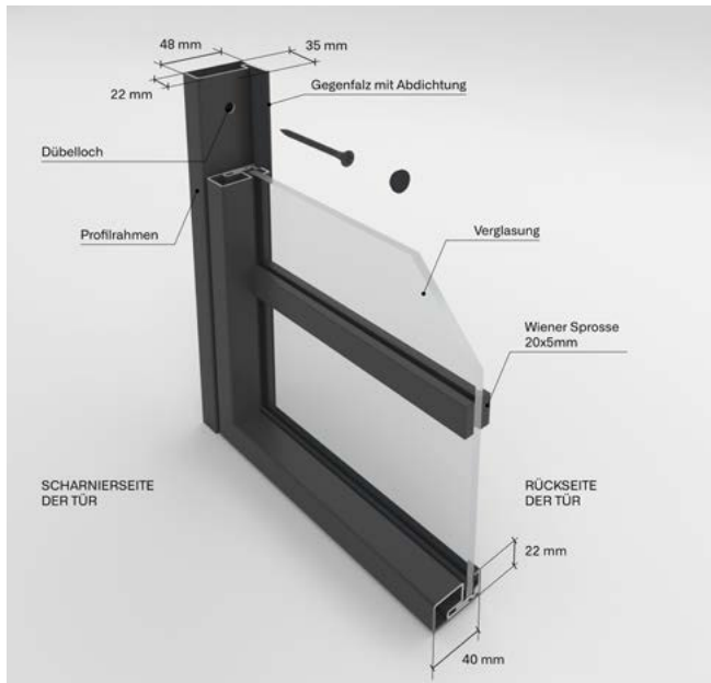
Rahmen- und Flügelquerschnitt mit Wiener Sprosse
