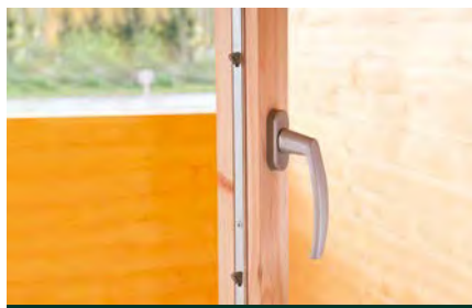
Dreh-/Kipp-Fenster mit 3-fach Verriegelung ab 34 mm
