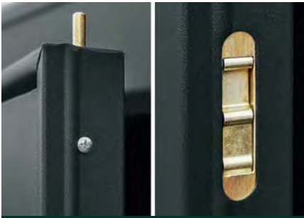
Feststellmechanik der 2-flügeligen Türen
