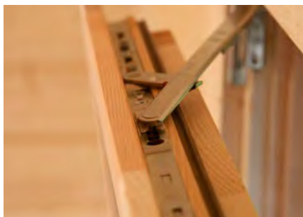
Dreh-/Kippbeschlag
